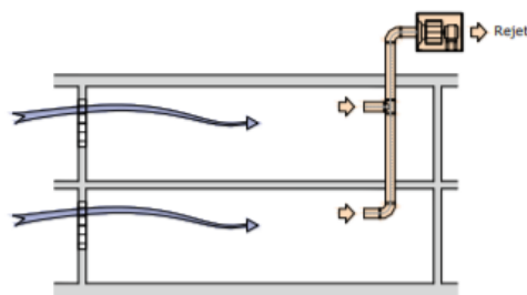
Figure 2 : surventilation simple flux en extraction
